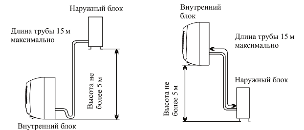
Схема установки
